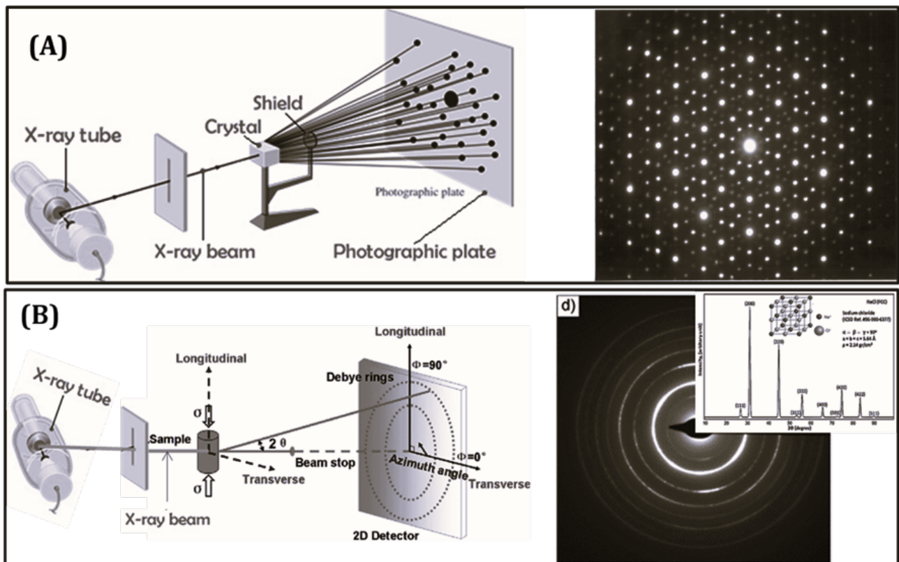
Hình 3: Sơ đồ nguyên lý của hiện tượng nhiễu xạ tia X trên tinh thể và ảnh nhiễu xạ: (A) mẫu đơn tinh thể và (B) mẫu đa tinh thể (ảnh ở góc là giản đồ nhiễu xạ tia X của mẫu)
