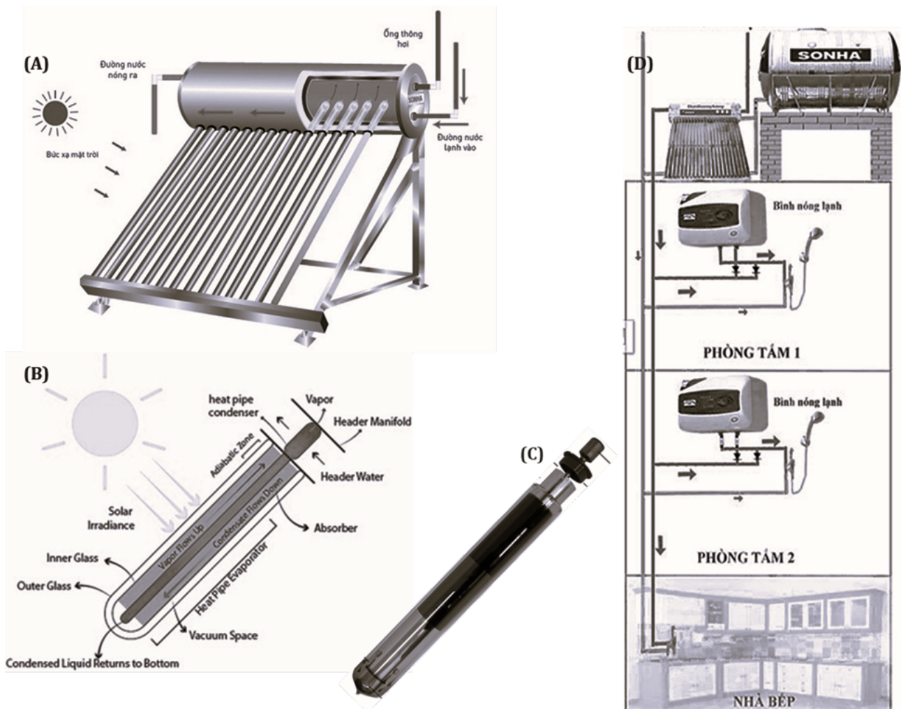
Hình 1: (A) Mô hình máy nước nóng năng lượng mặt trời; (B) Cấu tạo ống chân không ống nhiệt hiệu quả cao của máy nước nóng năng lượng mặt trời; (C) Ống nhiệt thực tế trên thị trường và (D) Sơ đồ lắp đặt thiết bị tới các phòng tắm và nhà bếp.
