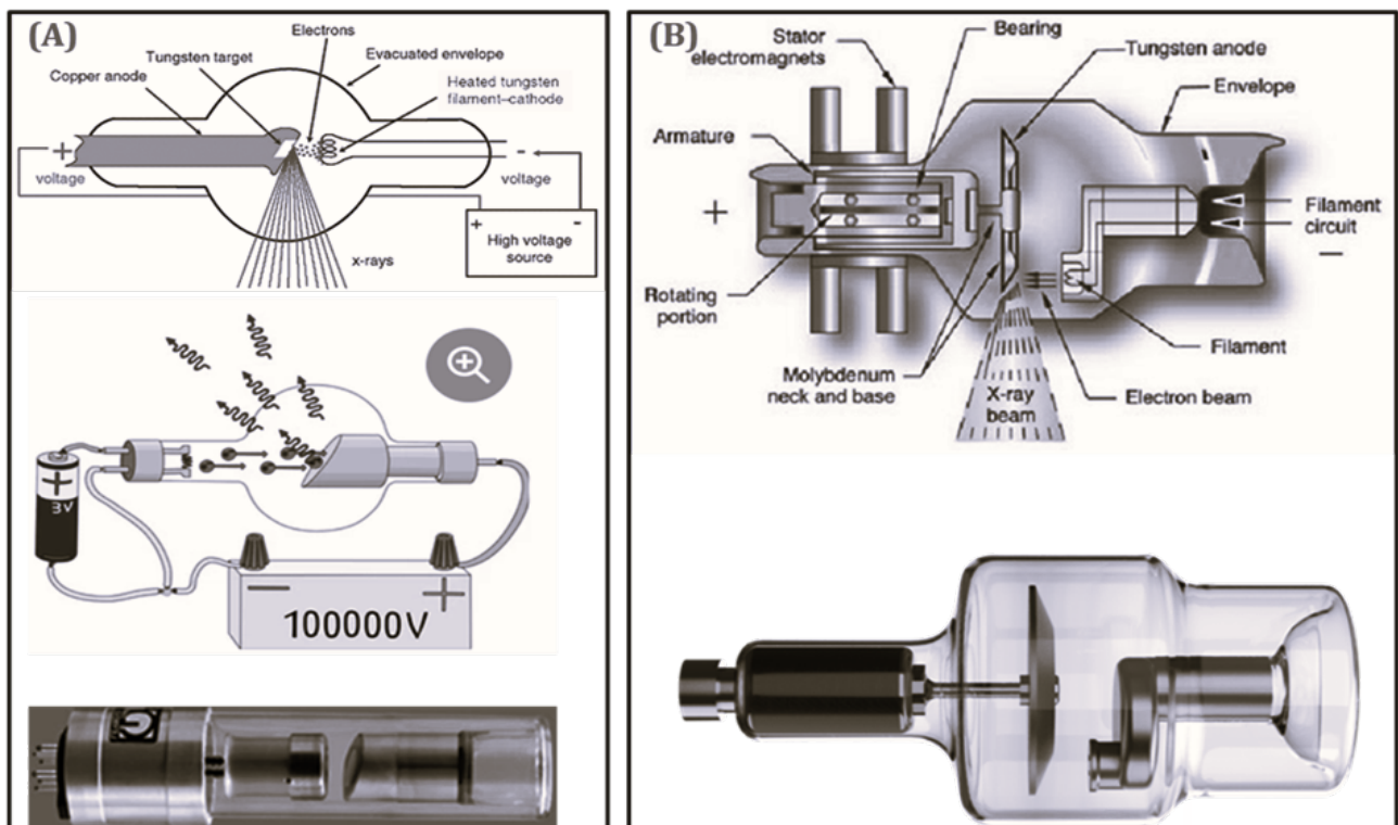
Hình 1: Cấu tạo của ống phát xạ tia X: (A) ống phát xạ tia X công suất thấp và (B) ống phát xạ tia X công suất cao.
