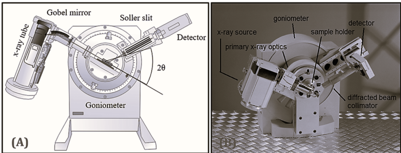
Hình 2: (A) Sơ đồ nguyên lý của máy đo nhiễu xạ tia X và (B) Máy đo nhiễu xạ tia X thực tế
